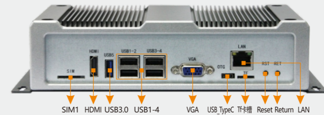
前面板接口
